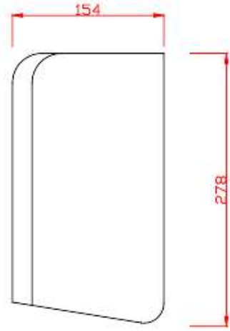
YAN GÖRÜNÜŞ
