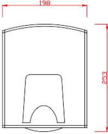
ÖN GÖRÜNÜŞ
