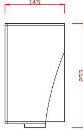
YAN GÖRÜNÜŞ
