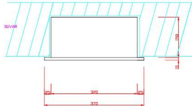
PLAN &lt;ANKASTRE SIVA ALTI&gt;
