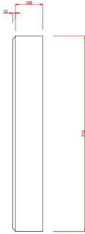
YAN GÖRÜNÜŞ
