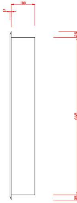
YAN GÖRÜNÜŞ
